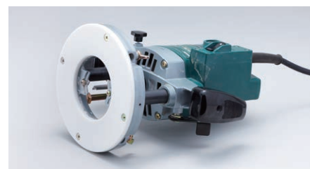
ベースプレートをコーリアン®にしたルーター
